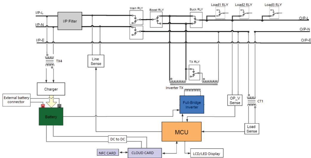
Figure 2. Schéma fonctionnel SMART1500LCDXNC
